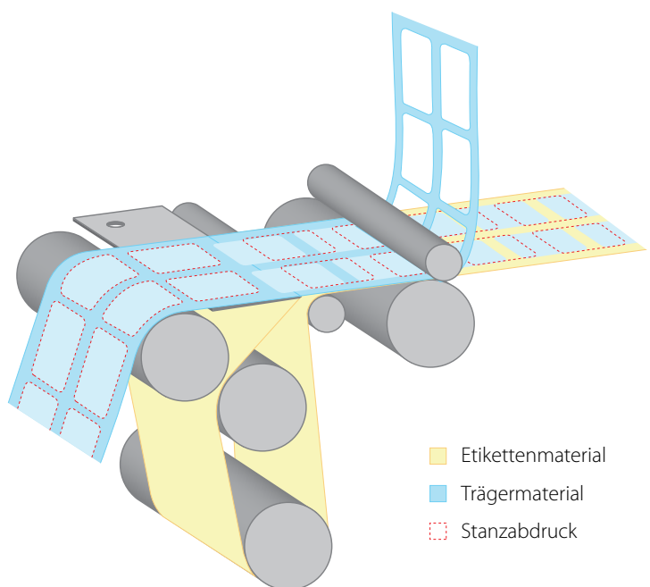
Schemadarstellung LabelShifter Plus
